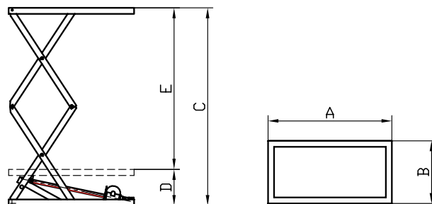
Massblatt Doppel-Scheren-Hebesystem
